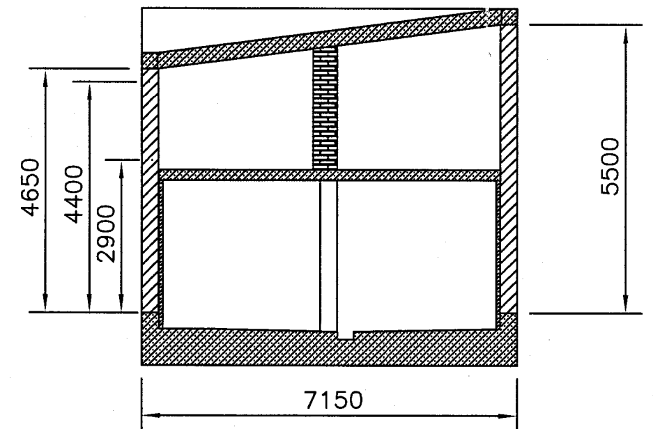
LEIKKAUS B-B POHJOISESTA
