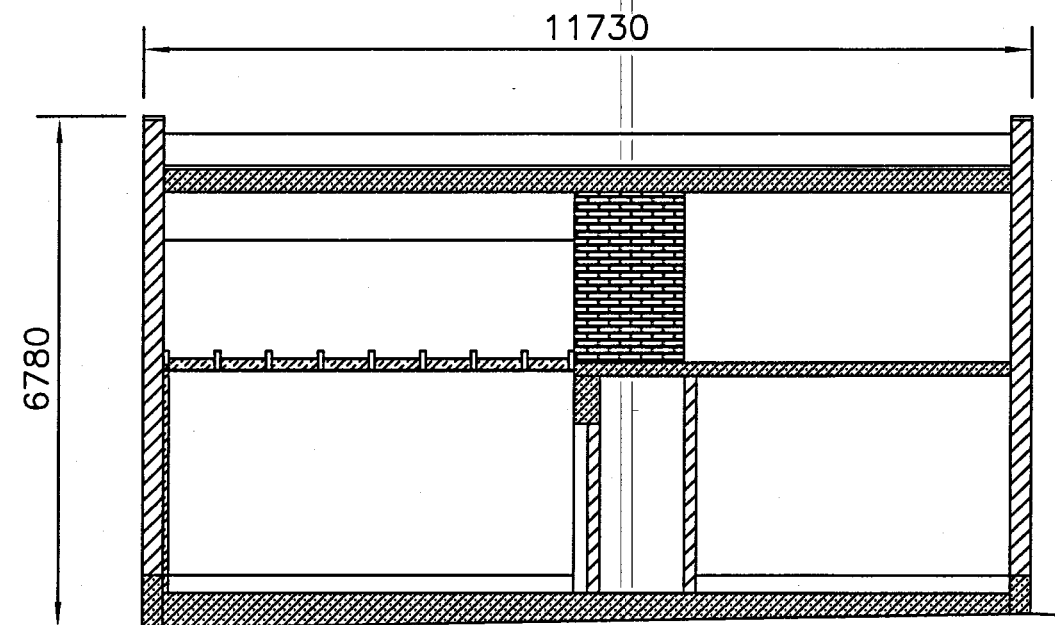
LEIKKAUS C-C IDÄSTÄ
